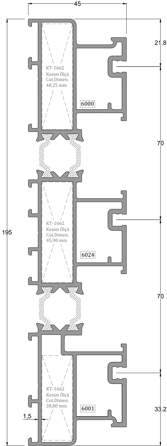
Üç Raylı Sineklikli Kasa Profili TRIPLE RAIL SCREENING FRAME PROFILE
